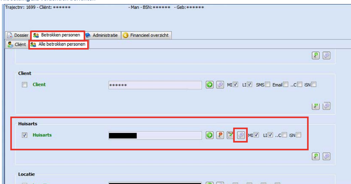
Afbeelding 2.1 Verzenden berichten
