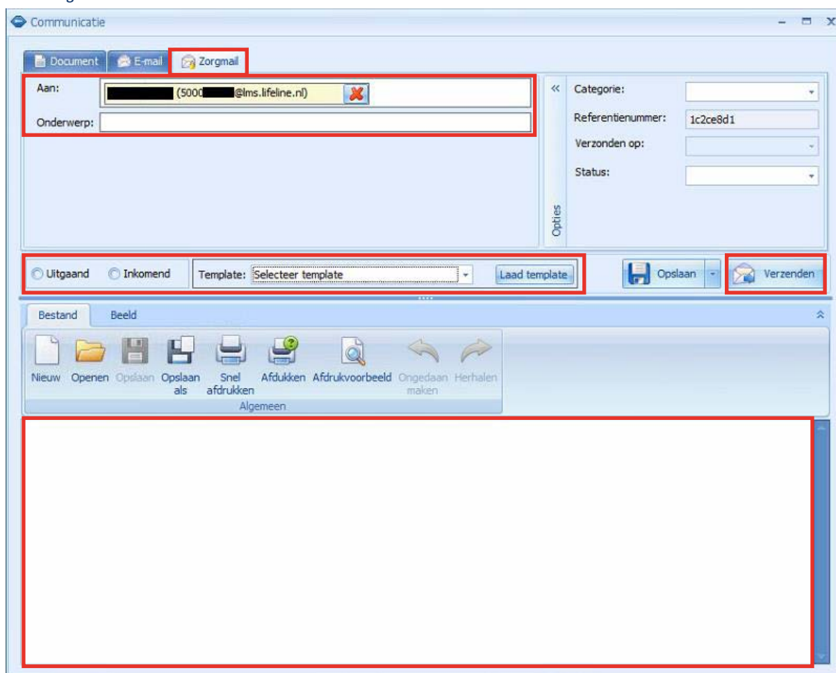
Afbeelding 2.2 Verzenden berichten
